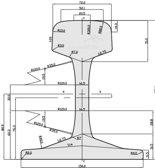
Figure 6: Profile of Standard UIC60 (EN 13674-1)
